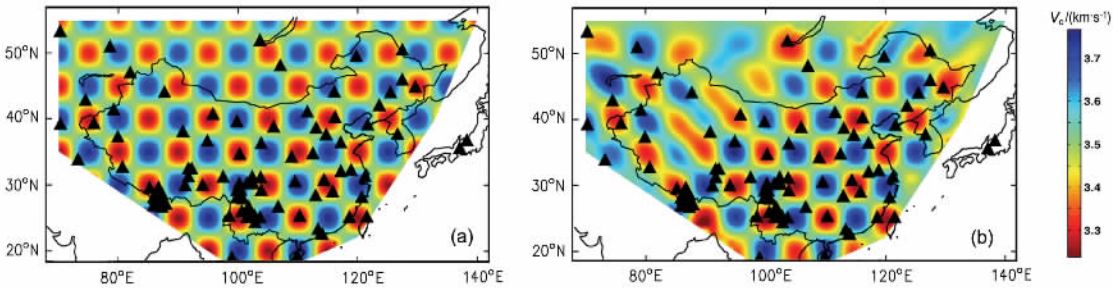
图4 40s周期时 5°×5°的检测板分辨率测试
